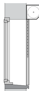
Enroulement extérieur
